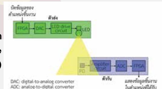
รูปที่ 2: โครงสร้างพื้นฐานของระบบส่งข้อมูลผ่านหลอดแอลอีดีส่องสว่าง
