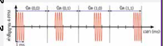
รูปที่ 3: สัญญาณข้อมูลแบบ 4-PPM (ไม่ได้แสดงบิตสำหรับ Synchronization)
